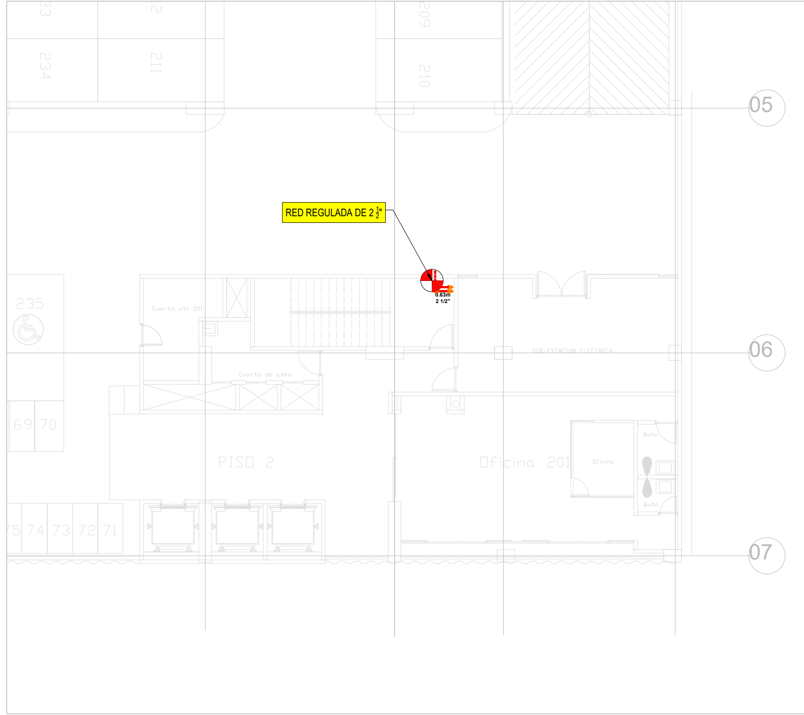
3 VISTA EN PLANTA PISO 2
